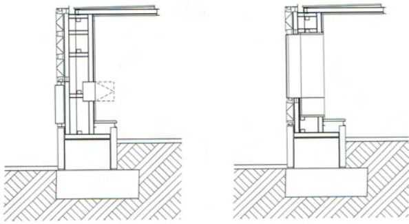
Fassadenschnitt mit Büchervitrine (links) und Sitznische (rechts)
